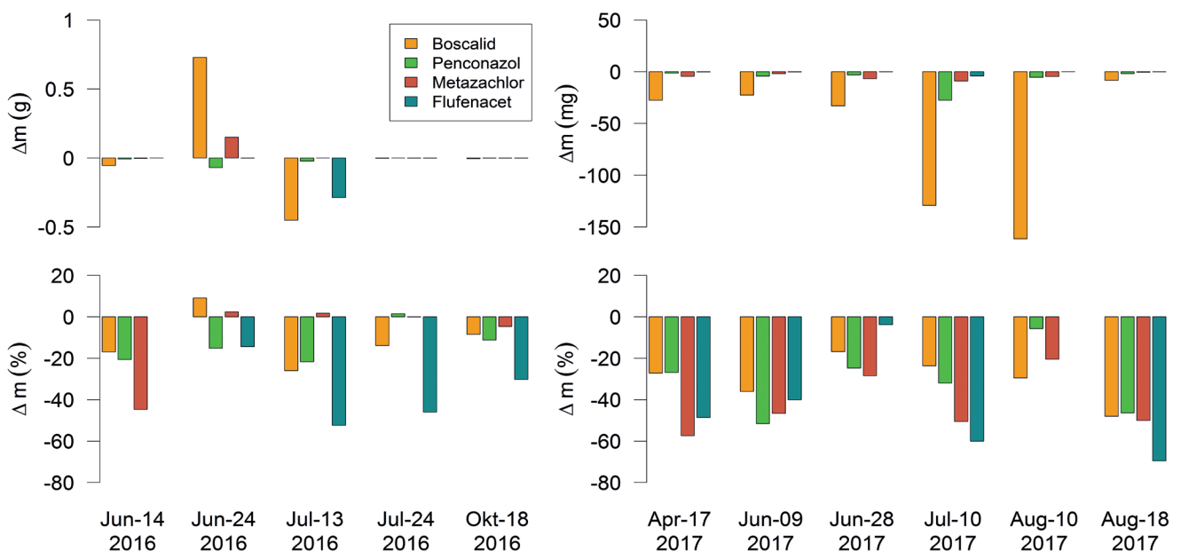
Abb. 3: Absolute und relative PSM-Massenbilanzen im Feuchtlächensystem bei Abflussereignissen 2016 (links) und 2017 (rechts)
