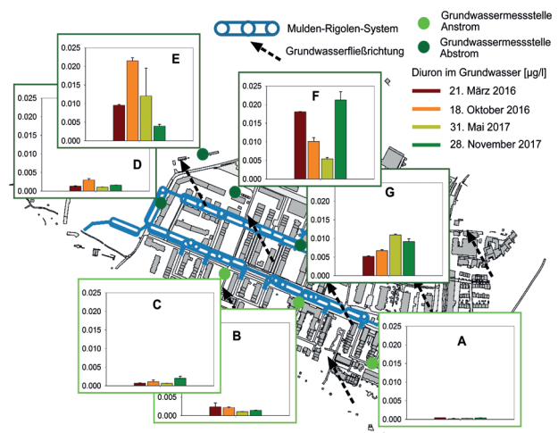
Abb. 4: Stichtagsbeprobung von Grundwasser im Umfeld eines Mulden-Ri- golen-Versickerungssystems; A-C Messstellen im Grundwasseranstrom, D-G: Messstellen im Grundwasserabstrom
